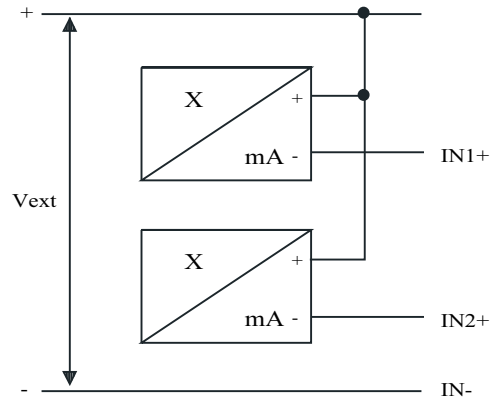
FIG. 4 TRASMETTITORI 4...20 mA 2 fili ALIMENTATI ESTERNAMENTE (Vext)
