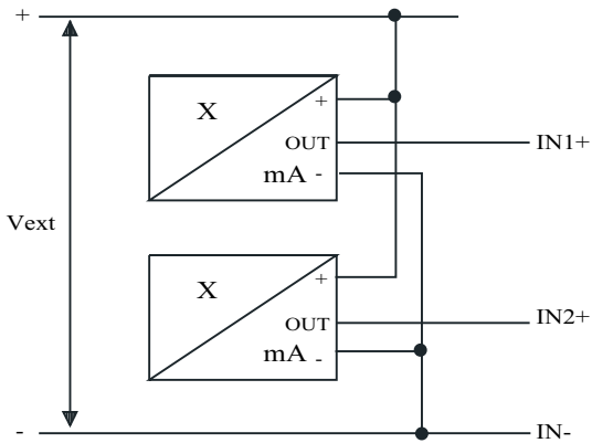
FIG. 5 TRASMETTITORI 4...20 mA 3 fili ALIMENTATI ESTERNAMENTE (Vext)
